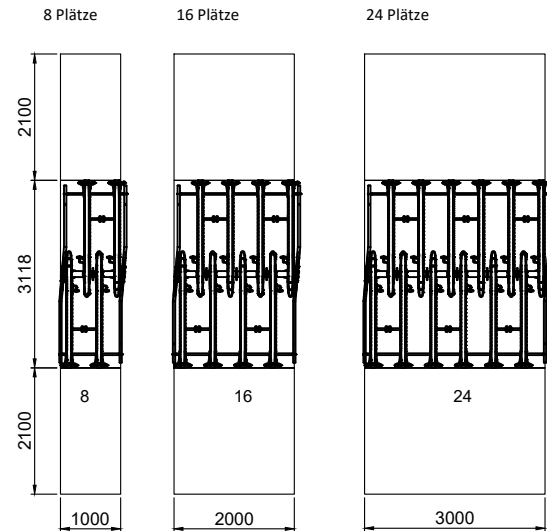
Easylift 500D, doppelseitig, Radabstand 500 mm
