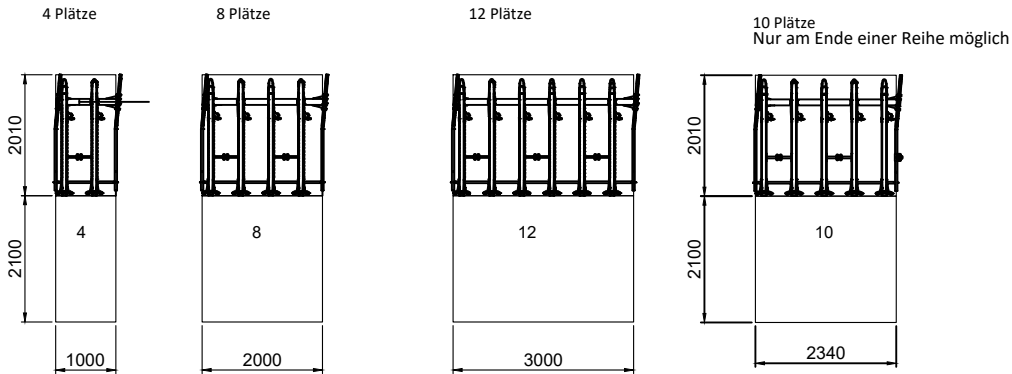
Easylift 500D, doppelseitig, Radabstand 500 mm
